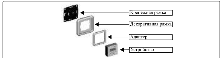
Рисунок 3. Крепление устройства
